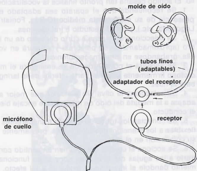
Enmascarador de Edimburgo para la corrección de la tartamudez.
